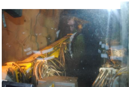
Att ensam köra en bormaskin på 1000 meters djup är vardag för gruvarbetarna i Renström. (Bild tagen inifrån hytten, därav speglingen i fotot)
